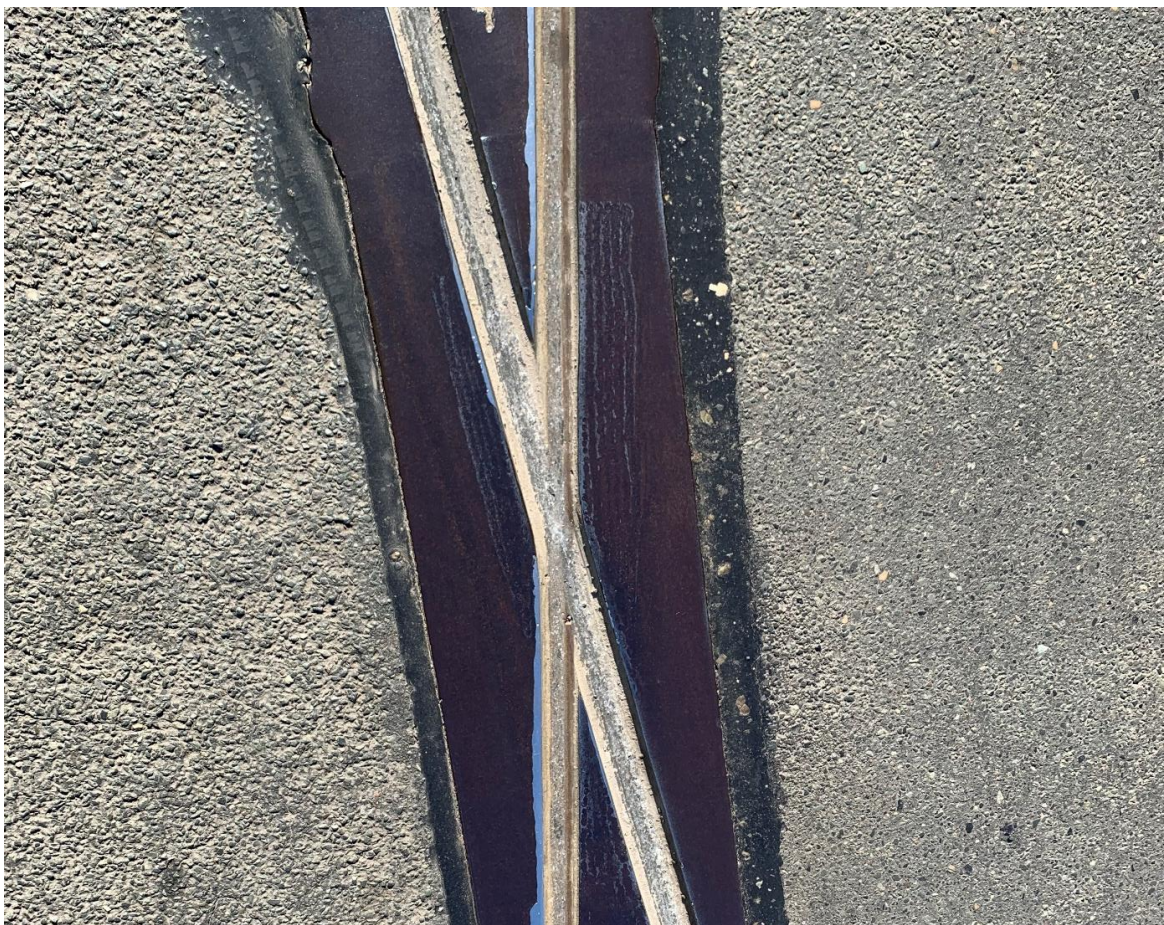
Abbildung 10: Verschleiß am Gleisdreieck Pirckheimerstraße
